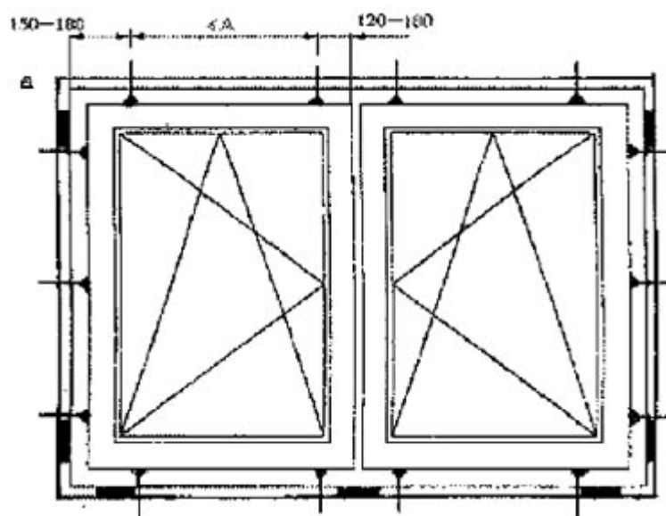
Рисунок В.1 – Примеры расположения опорных (несущих) колодок и крепежных деталей
