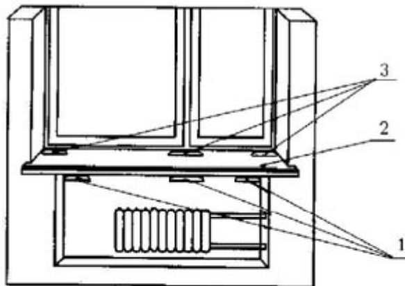
Рисунок А.16 – Узел углового соединения оконных коробок
