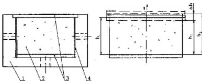
Рисунок 4 – Схема приспособления для испытания монтажных швов на деформационную устойчивость
