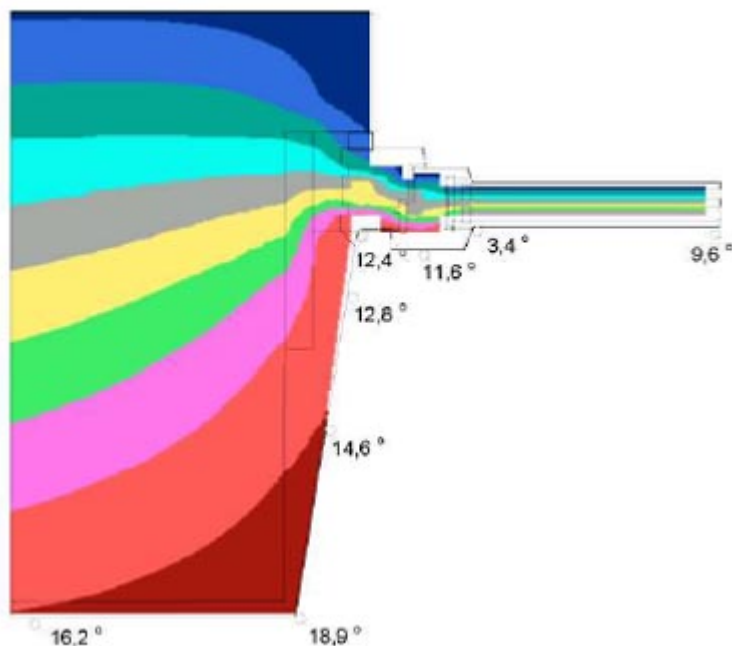
Рисунок Г.3 - Результаты расчета распределения температур по узлу примыкания оконного блока из клееной древесины к стене из полнотелого кирпича
