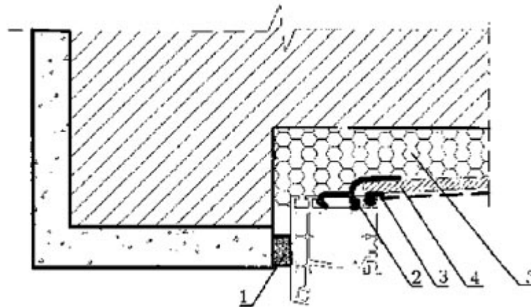
Рисунок А.12 – Монтажный шов в узле примыкания оконной коробки из профиля ПВХ (127 мм), подоконника и отлива в проеме однослойной стены
