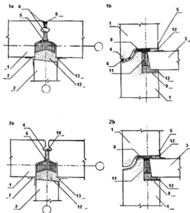
Варианты конструкций стыков «открытого» и «закрытого» типов: Рис. 1а. Вертикальный стык «закрытого» типа Рис. 1б. Горизонтальный стык «закрытого» типа Рис. 2а. Вертикальный стык «открытого» типа Рис. 2б. Горизонтальный стык «открытого» типа
